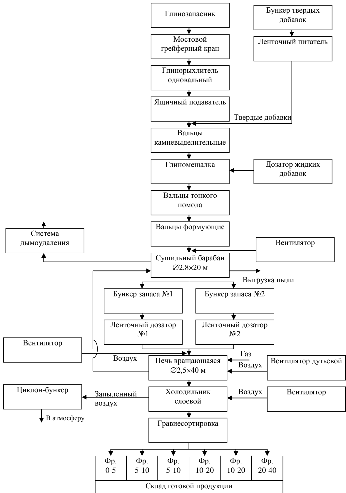
Рис. 1 Принципиальная схема комплекса
